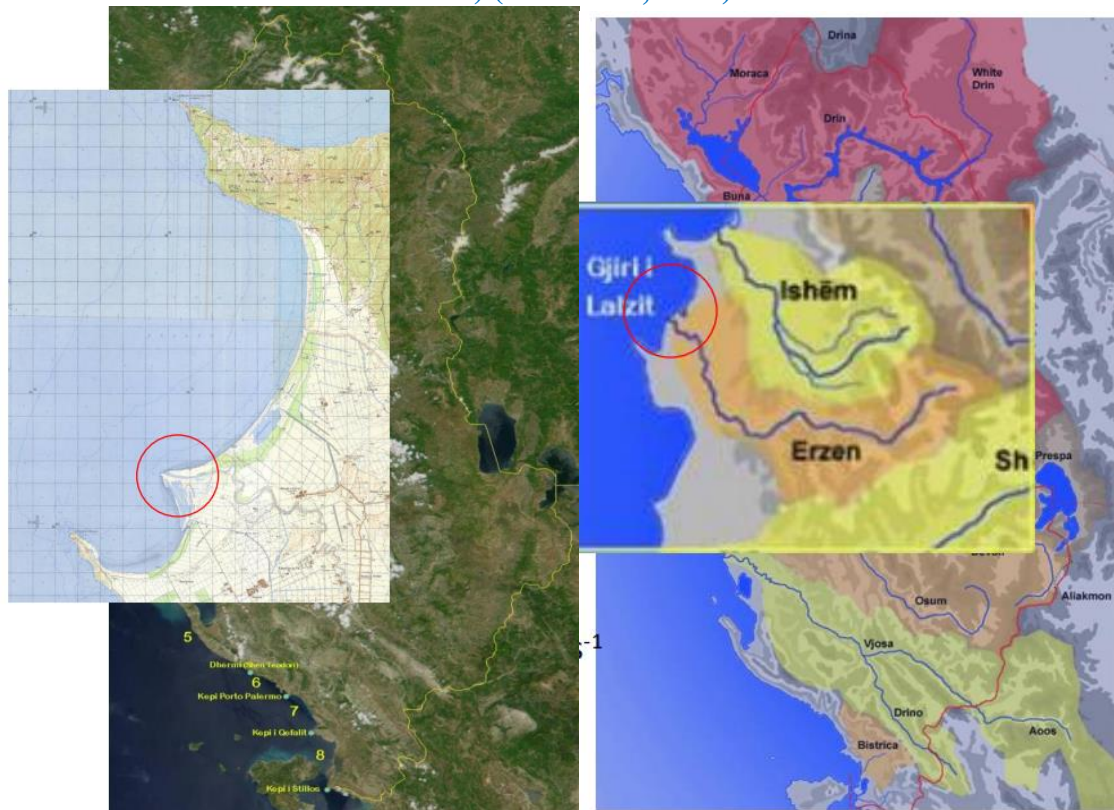
Figura 6 - Prerja e kanalit dhe erozioni bregdetar në lumin Erzen –Gjirit i Lalzit (1984 – 2015) (G. Zolezzi, 2019)
